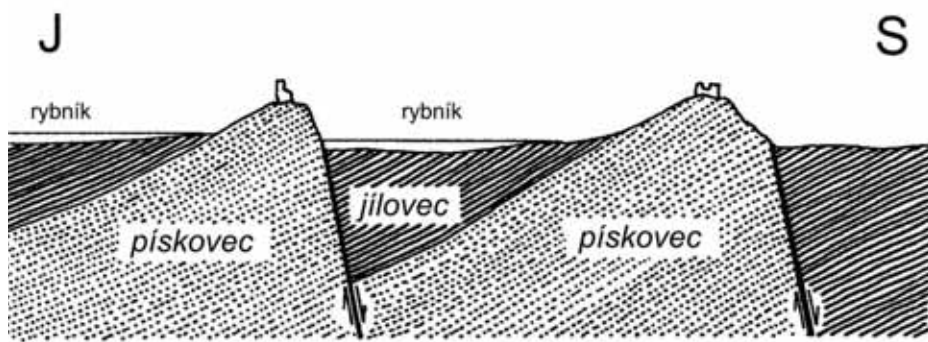
Obr. 1. Příčný řez geologickým podložím Holanských rybníků (schéma podle Bruno Müllera).
